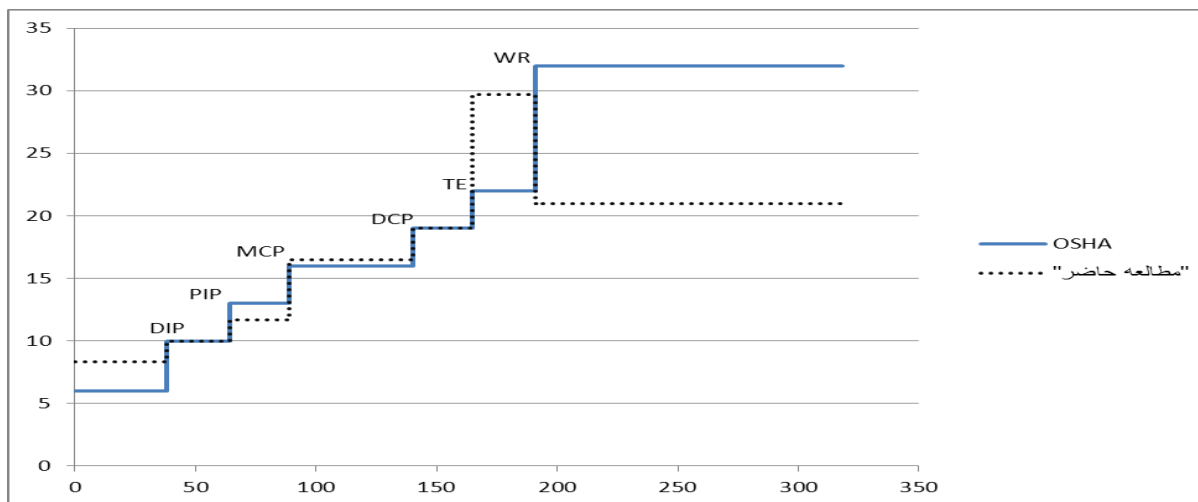
شکل ۳: مقایسه حفاظ (ماشین‌آلات)، پیشنهادی و استاندارد OSHA. DIP = انتهای‌ترین مفصل انگشت وسط از کف دست، PIP = نزدیک‌ترین مفصل انگشت وسط به کف دست، MCP = کف دستی (متاکارپال)، DPC = چین کف دستی، TE (CMCP) = برآمدگی قسمت گوشتی کف دست در قاعده شست، WR = مچ
